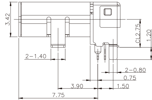
A-A SCALE 1:1
