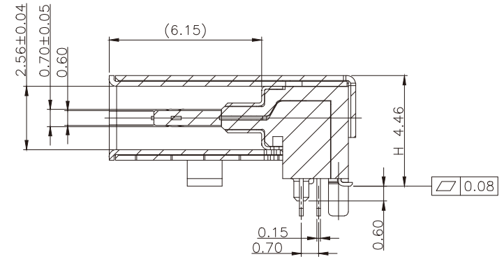
A-A SCALE 1:1
